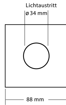
Oberteil quadratisch
