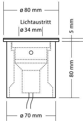
Oberteil bodeneben
