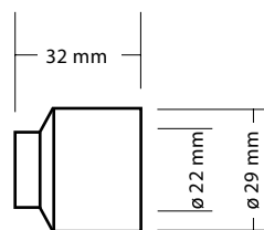
2 Scheinwerfer-Vorderteil
