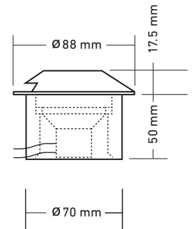
Kurz HL-LED
