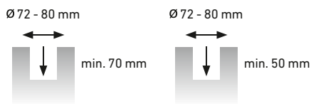
Winkelspot kurz
