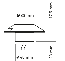
Effekt-LED
