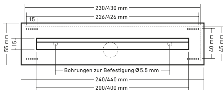
Down Light, Frontansicht
